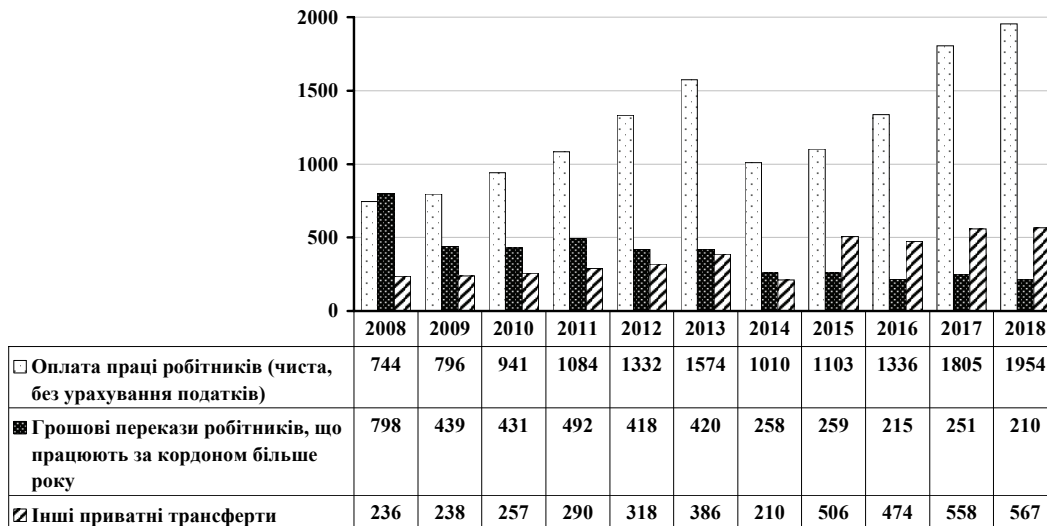
Рис. 6. Динаміка обсягів грошових переказів в Україну, млн дол. США
